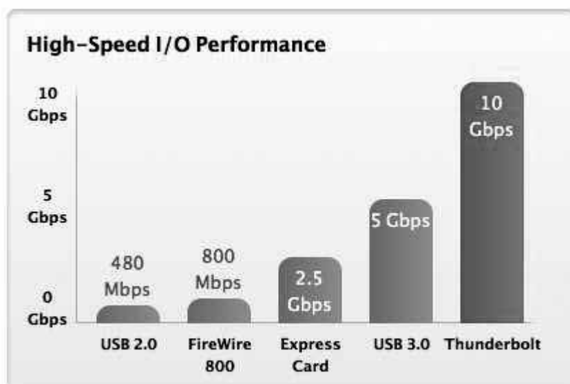
圖二：高頻連接器傳輸速度
